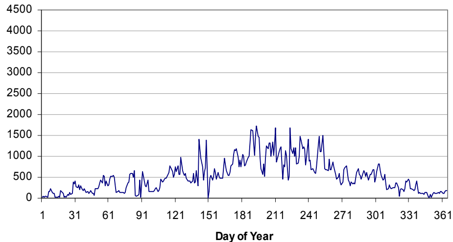
NOBS 2000 Vapor Pressure Deficit (Pa)
