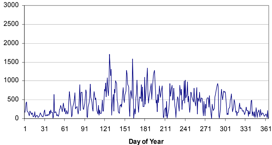
HARV 2000 Vapor Pressure Deficit (Pa)
